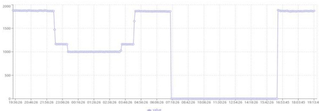
Slika 4 Režim rada javne rasvjete
